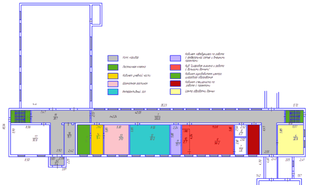
План 2 этажа Схема функционального зонирования
